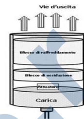
Schema generatore di aerosol
