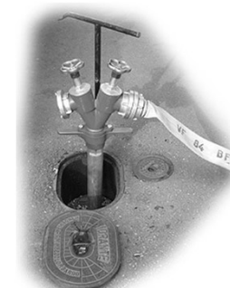
Idrante sottosuolo
