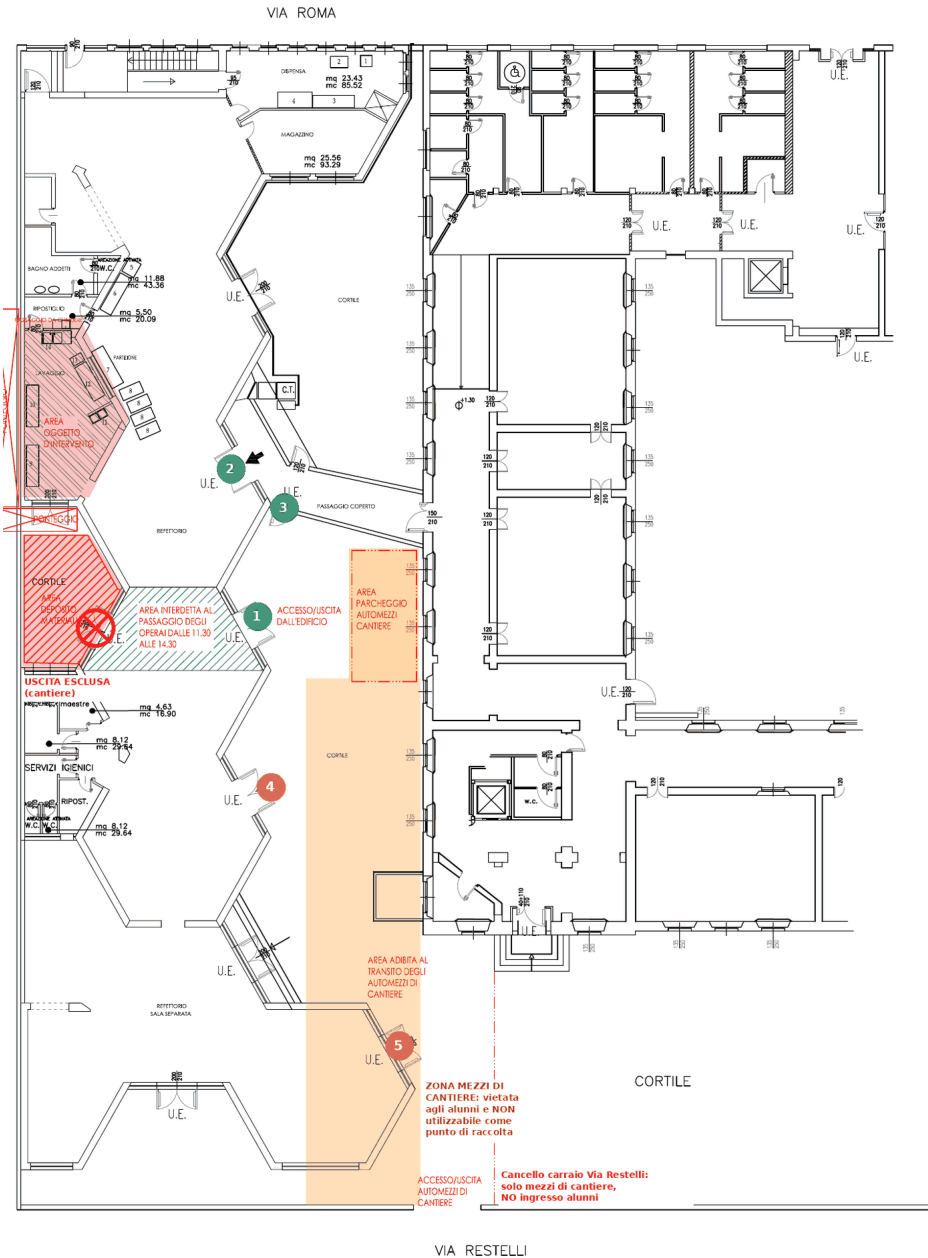
PLANIMETRIA TEMPORANEA DI EMERGENZA - Addendum rev.0 del 05/10/2026 Plesso G. Deledda - valida dal 09/10/2026 fino alla riconsegna delle aree Base: planimetria di cantiere CSE agg. 23/09/2026
