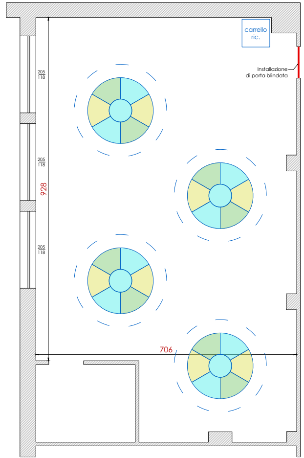
Secondaria Boezio - Piano Terra: Innovation Lab multifunzionale (stato di progetto)
