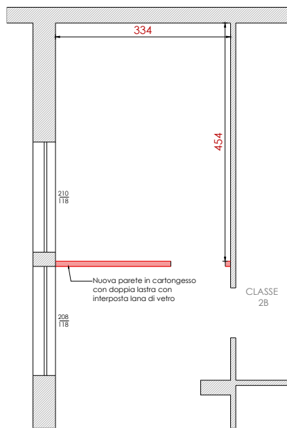
Secondaria Boezio - Piano Terra: Spazio inclusivo polifunzionale (stato di confronto)
